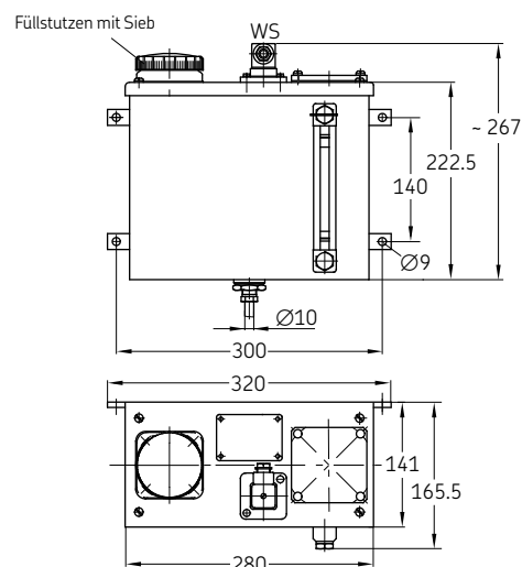
Metallbehälter, 6 Liter
