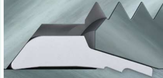
Doppelkantenschneidring-Verschraubung
