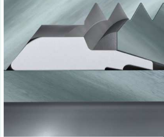
Doppelkantenschneidring-Verschraubung vor dem Anziehen
