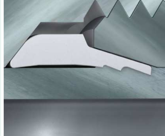
Doppelkantenschneidring-Verschraubung nach dem Anziehen
