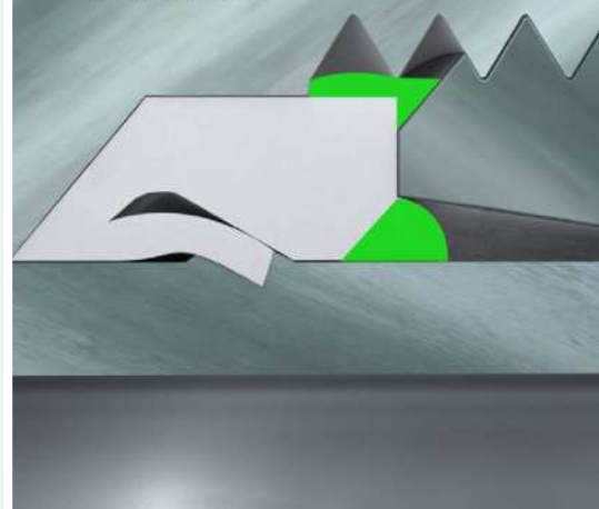
Verschraubung mit Schneidring und Weichdichtung nach dem Anziehen
