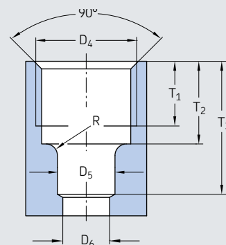
Senkungen für die lötlöse Rohrverbindung (DIN 3854/DIN 3862)
