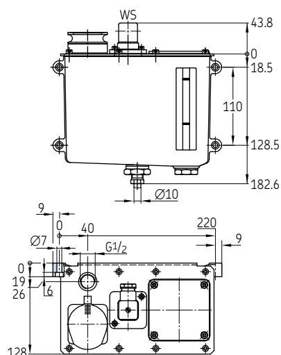
Metallbehälter, 3 Liter
