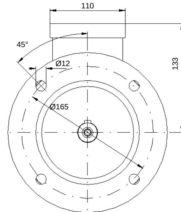
Kabelabgang / cable outlet
