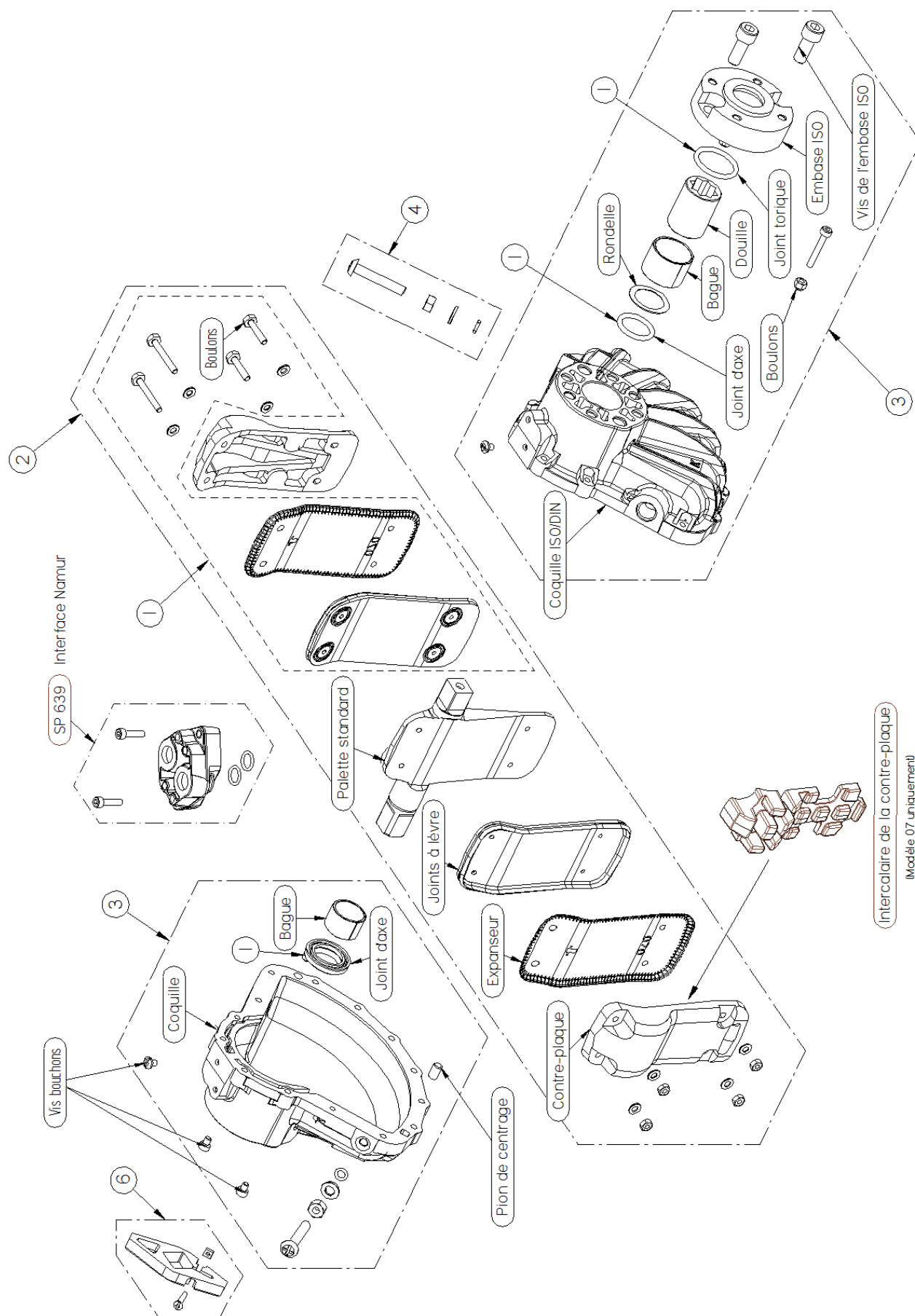
FIGURE 6 . VUE ECLATEE TYPIQUE D'UN ACTIONNEUR ISO/DIN
