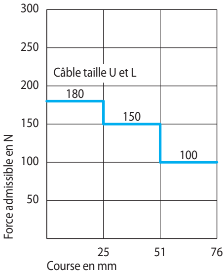
Force de traction avec série 775 - V1
