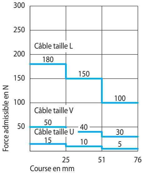
Force de traction avec série 283 et 275 - V1
