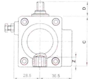
T - PA 40 CE Kesit detayı
